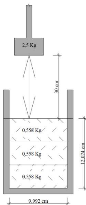
Obr. 7 – Schéma PS + hmotnost zeminy na jednu vrstvu
